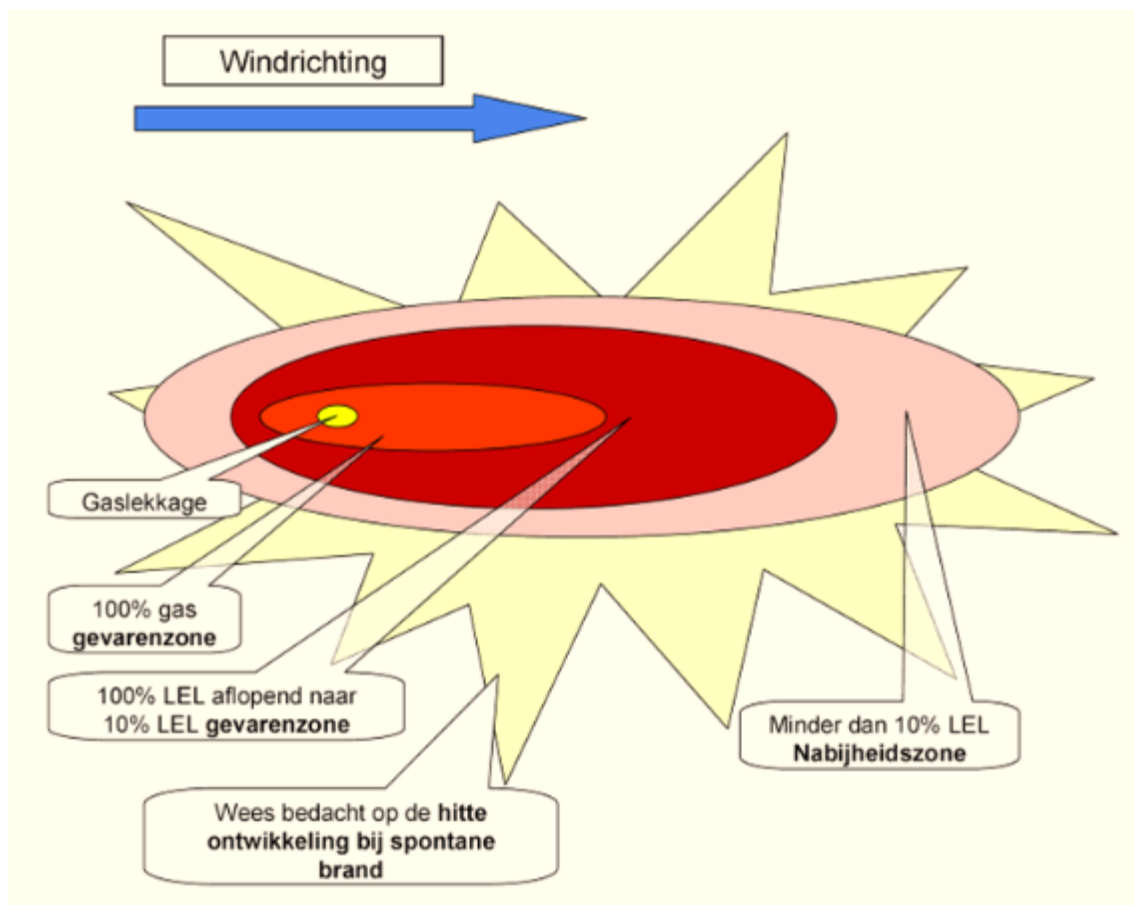
Figuur – Gevarenszone en nabijheidszone bij een groot gaslek.
