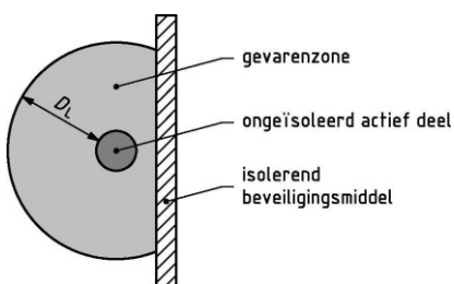
Figuur 2 – Gevarenzone bij gebruik van een isolerend beveiligingsmiddel.
