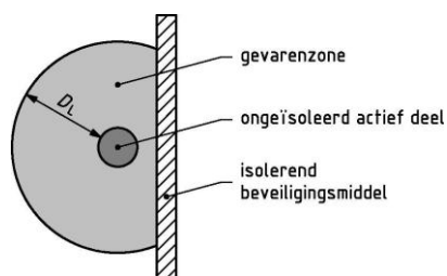
Figuur 2 – Gevarenzone bij gebruik van een isolerend beveiligingsmiddel.
