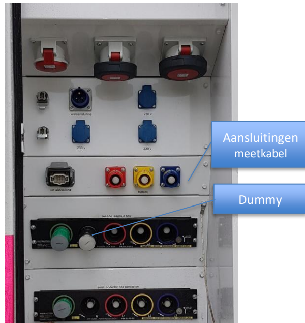
Foto 1: Aansluitboxen aggregaat
